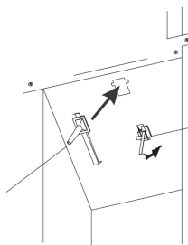
Der „Wassertank voll“ - Absperrschalter ist niedergedrückt, wenn das Ablaufrohr für kontinuierliche Entwässerung befestigt ist.
